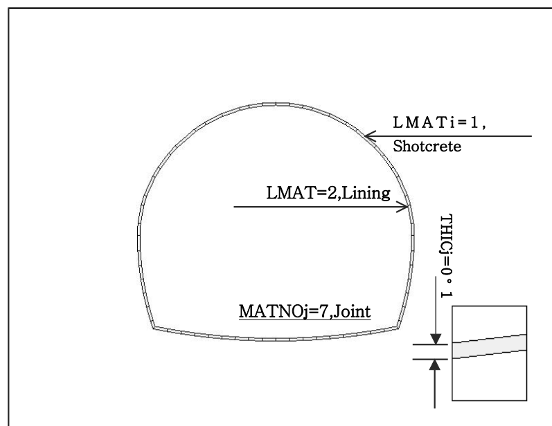
그림 5. 터널 Shotcrete / Lining Interface
